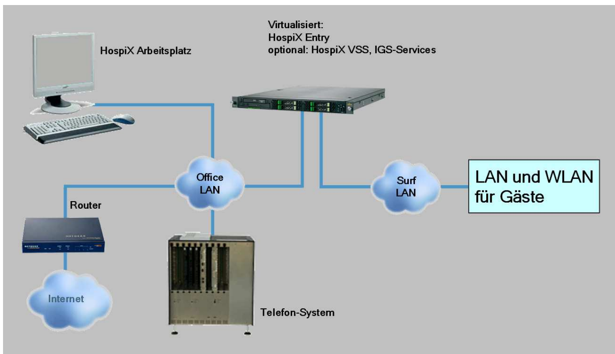
Beispiel: Konfigurationsschema
